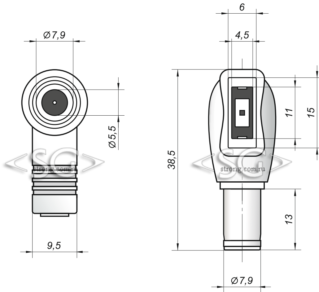
Вид А
