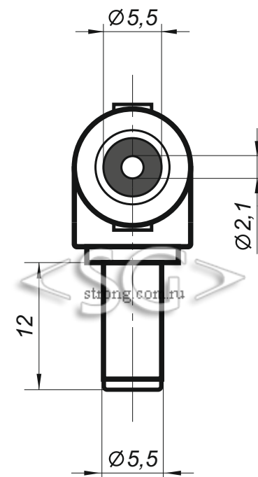
Вид В
