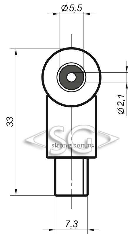
Вид В
