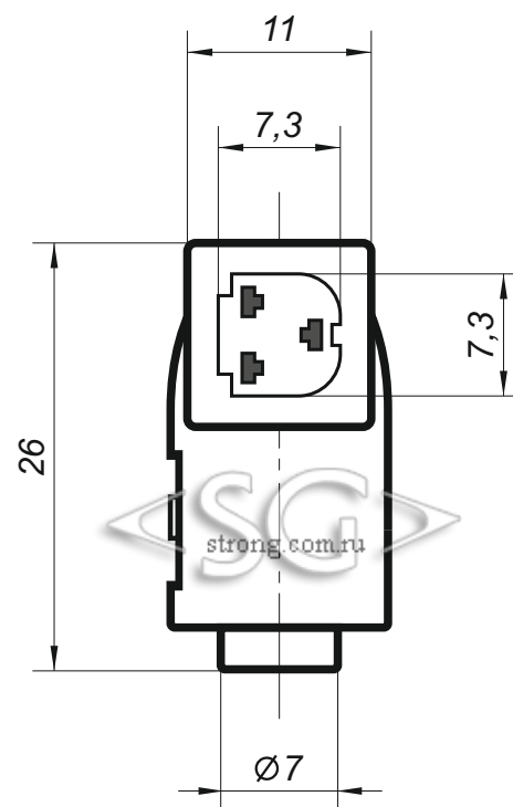
Вид А
