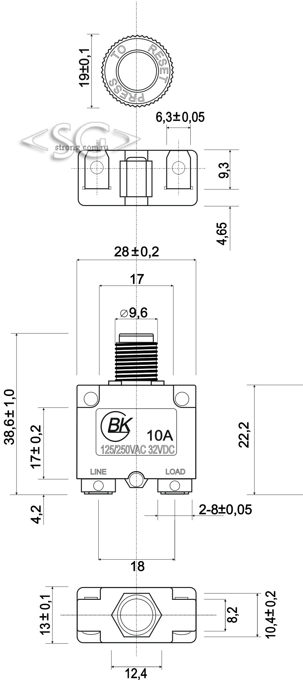
Вид А
